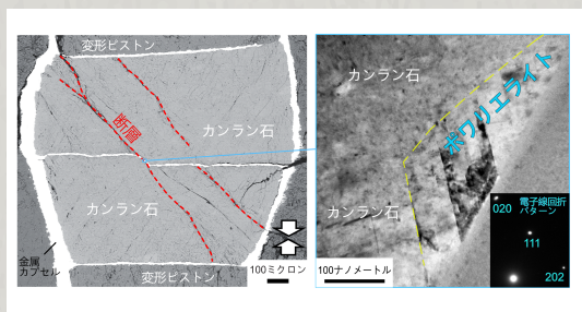
図：15.4万気圧、850°Cの実験環境下にて上下方向からカンラン石試料を押しつぶした際に形成された断層。いずれも電子顕微鏡で撮影。左側：試料全体の写真。試料を横断する断層（赤破線）が見られる。右側：カンラン石の結晶構造が変形することで生成したポワリエライト。図右下は当該結晶がポワリエライトであることを示す、電子線回折パターン像。100マイクロは1ミリの10分の1。100ナノメートルは1ミリの1万分の1。
